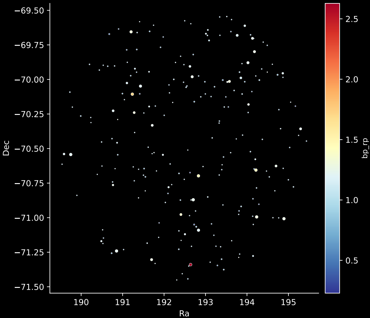
GALAH DR4 Field: [7133] Stars: 228
