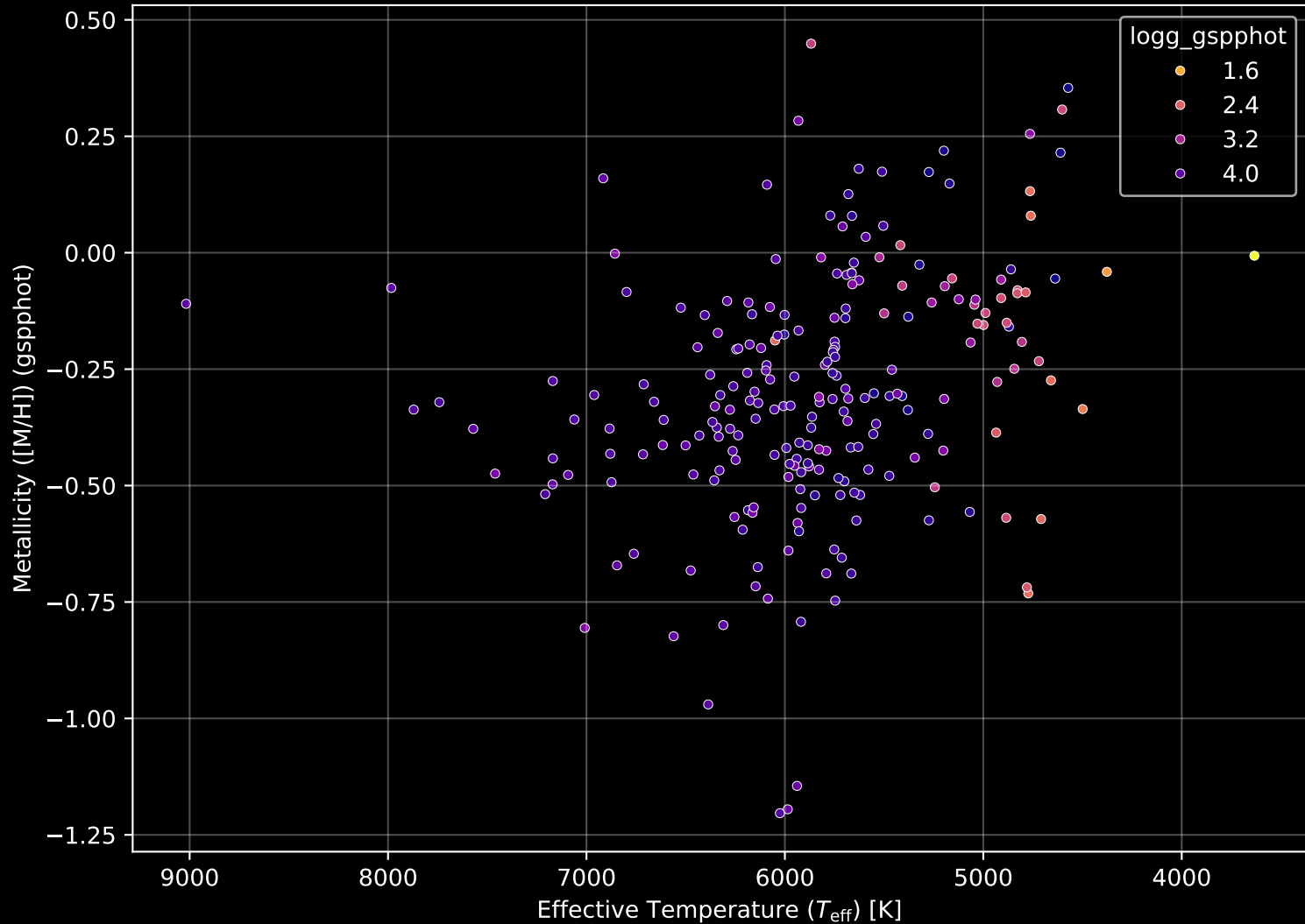
GALAH DR4 Field: [7133] Stellar Population Parameters (n= 228)
